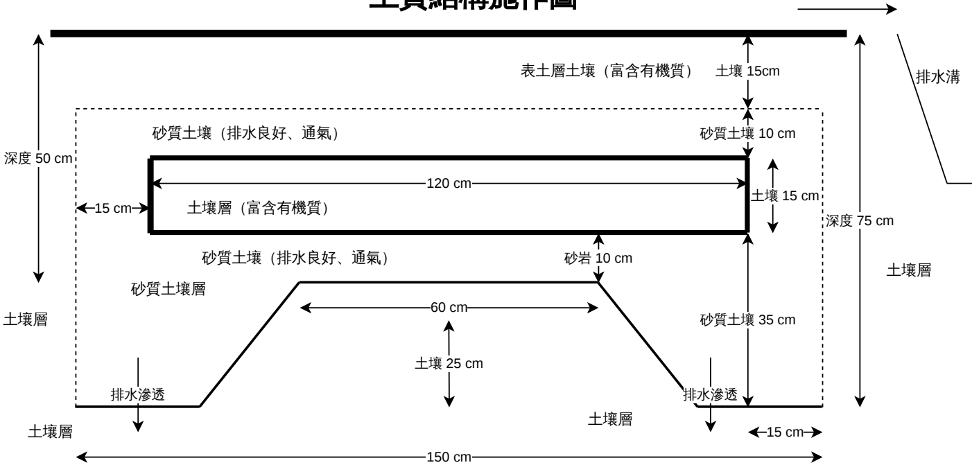
土質結構施作圖
